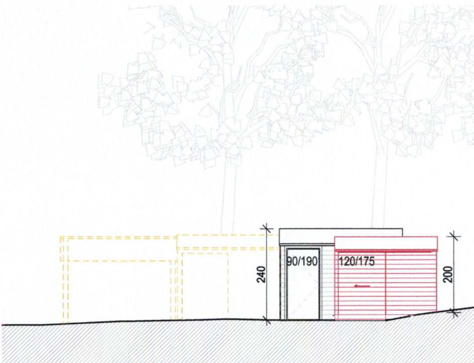
Coupe A3
