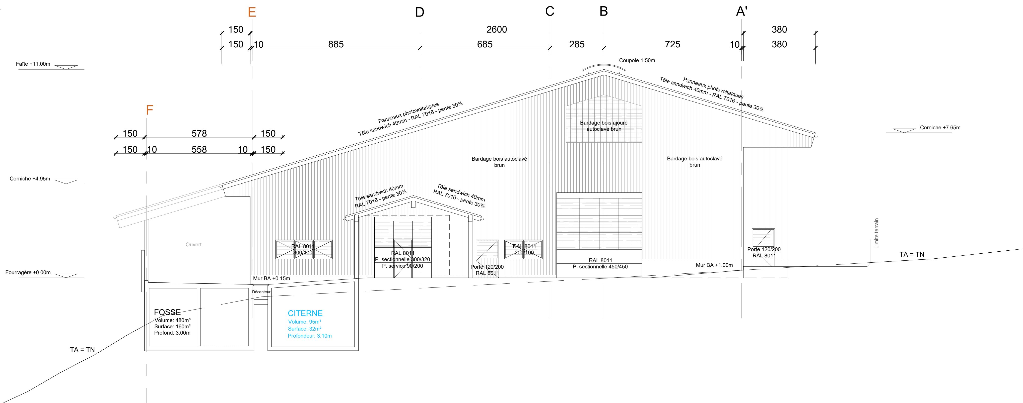
FACADE NORD-EST
