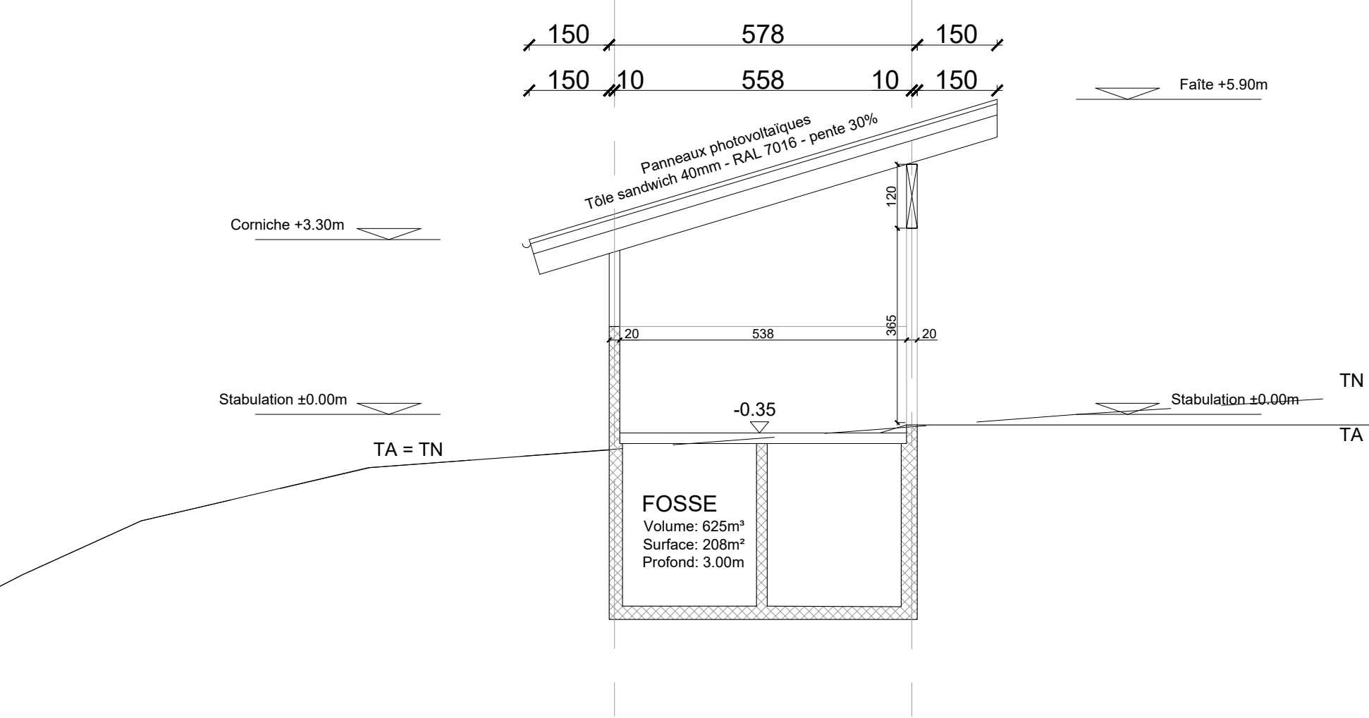
COUPE C-C
