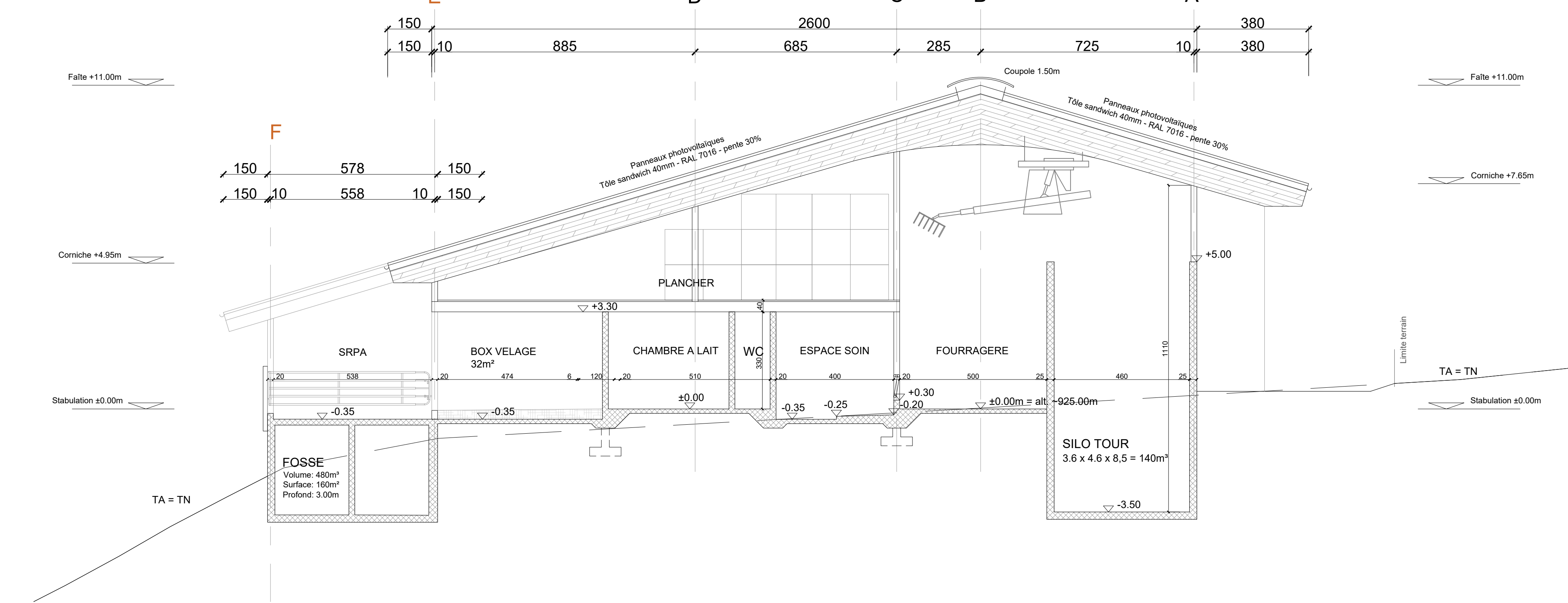
COUPE B-B
