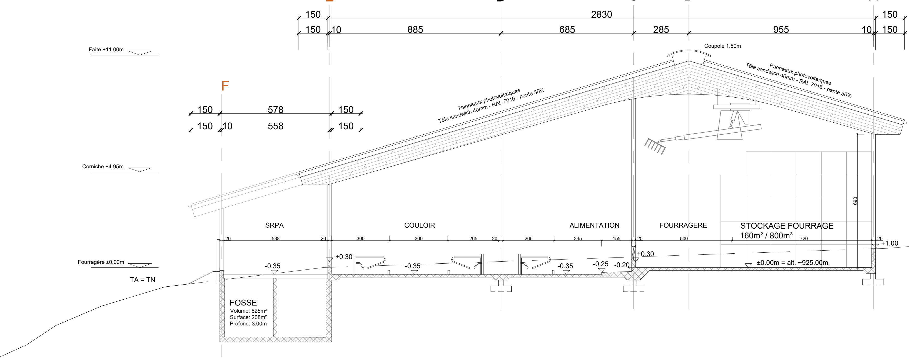
COUPE A-A
