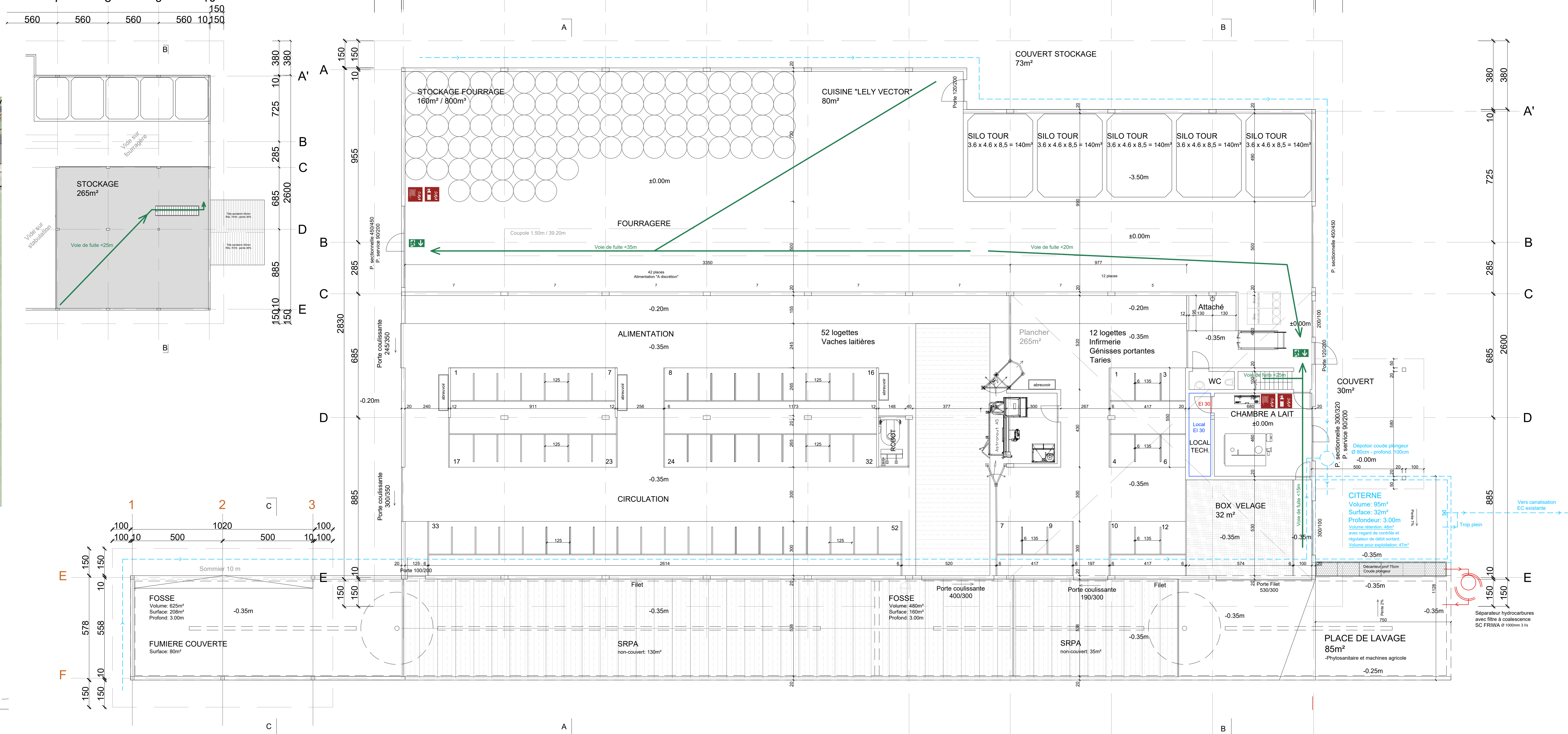
PLAN ETAGE 1:200
